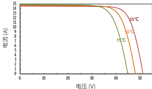
JT575SGt 不同温度下的IV曲线
