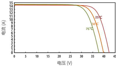
JT470SHt 不同温度下的IV曲线
